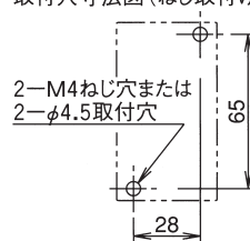
取付穴寸法図(ねじ取付けの場合)
